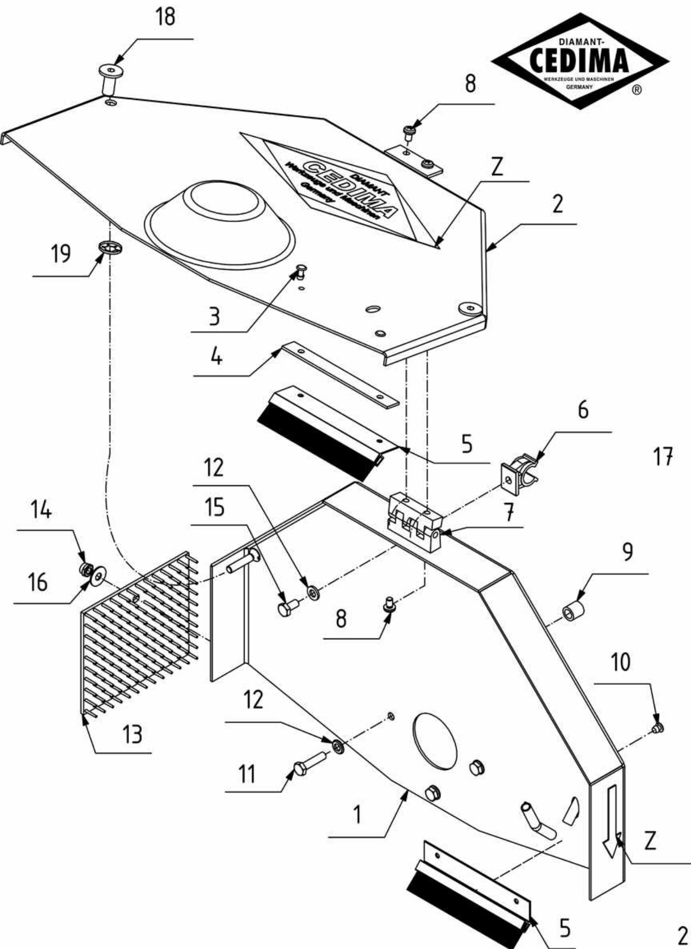
Blattschutz kmpl. Blade cover cmpl. CTS-57G Pos.WA
